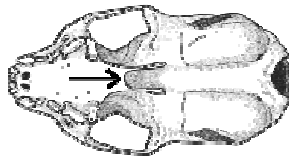
M. erminea
